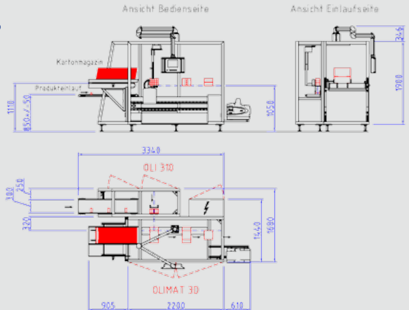
Plan d'ensemble oli 310 avec olimat 3D
